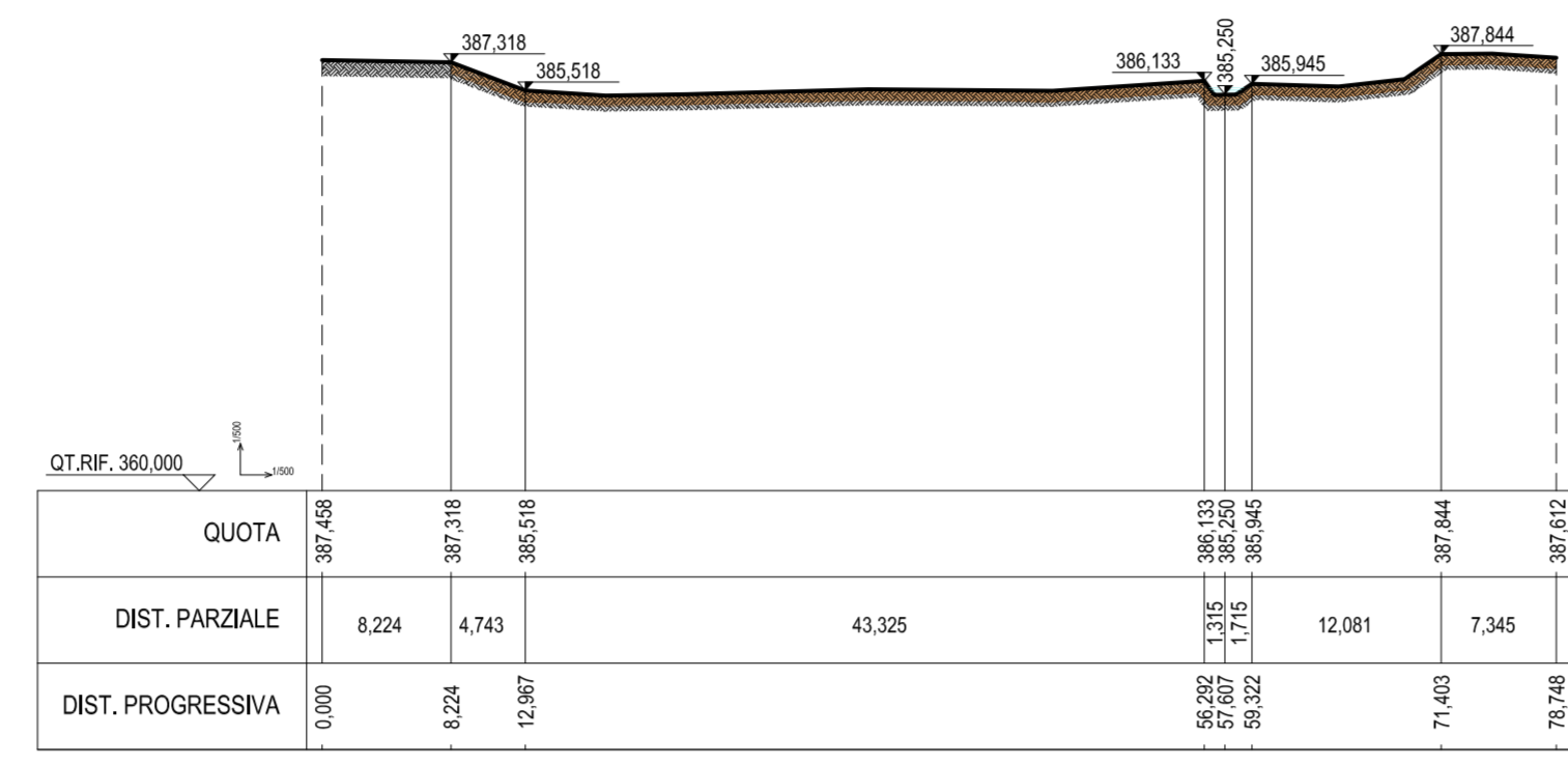
SEZIONE N. : 1-1'
