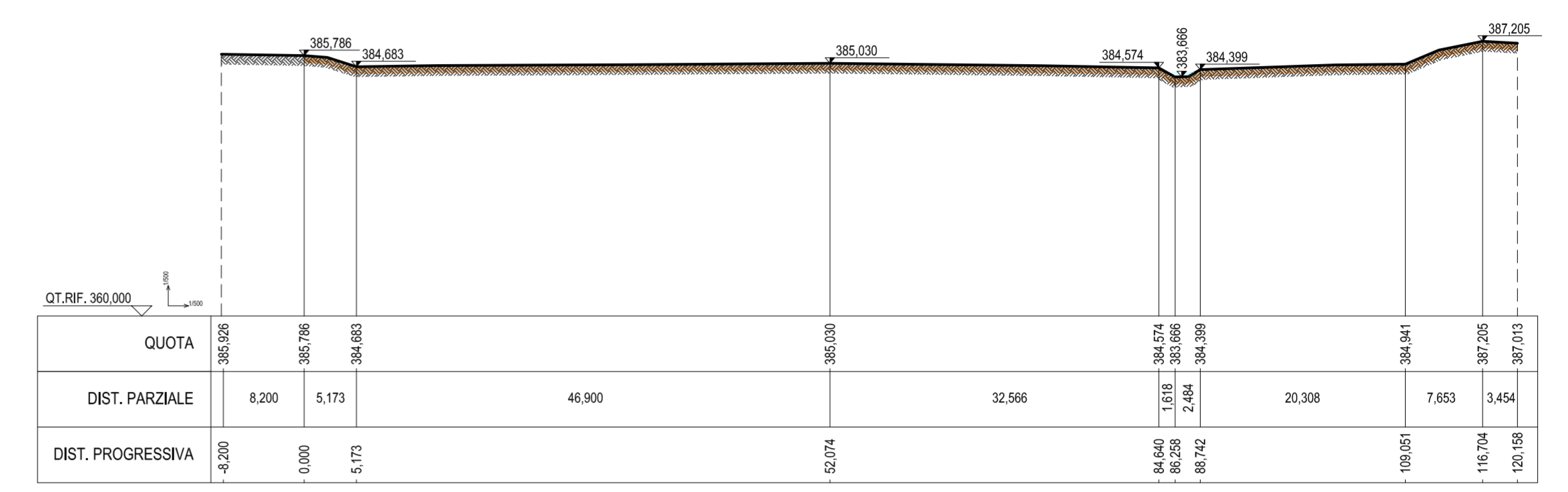
SEZIONE N. : 2-2'
