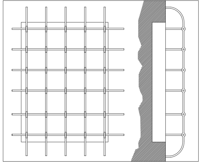
facciata n. 210 - a maglia ortogonale
