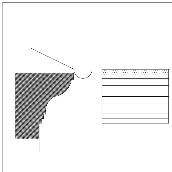
facciata n. 55 - a guscio
